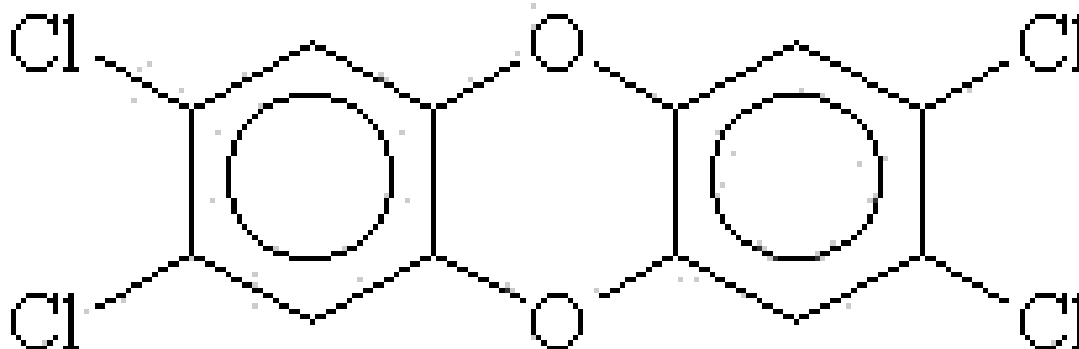
2,3,7,8-тетрахлордibenзо-п-диоксин
